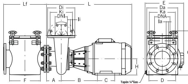
OPT-FD750 / FD1000 / FD1250
