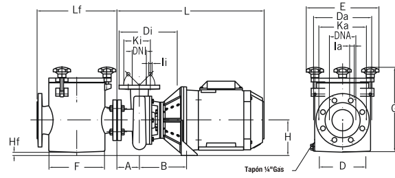
OPT-FD750 / FD1000 / FD1250
